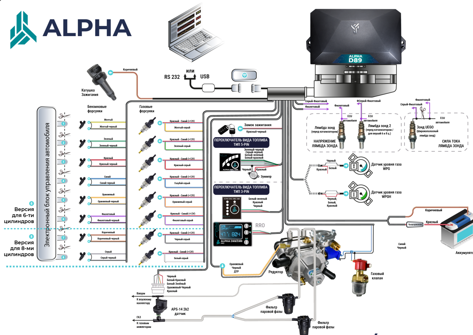
МОНТАЖНАЯ СХЕМА ALPHA D69 / D89
